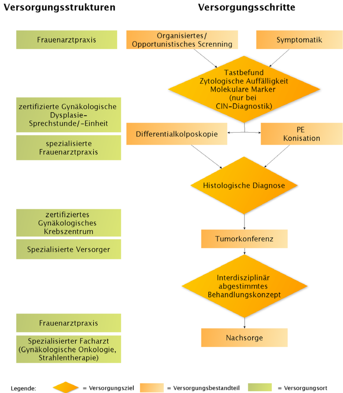
Abbildung 1: Konsentierter Versorgungsalgorithmus
